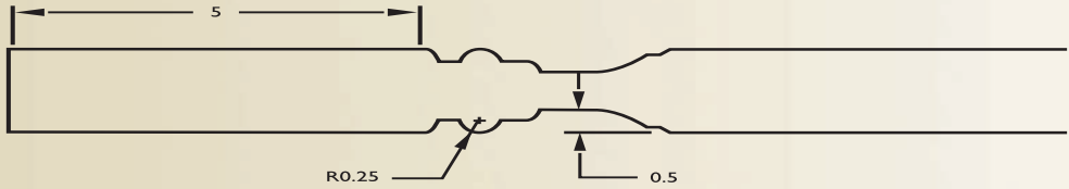
Optional Flush Molding Specify "with Flush Molding"
